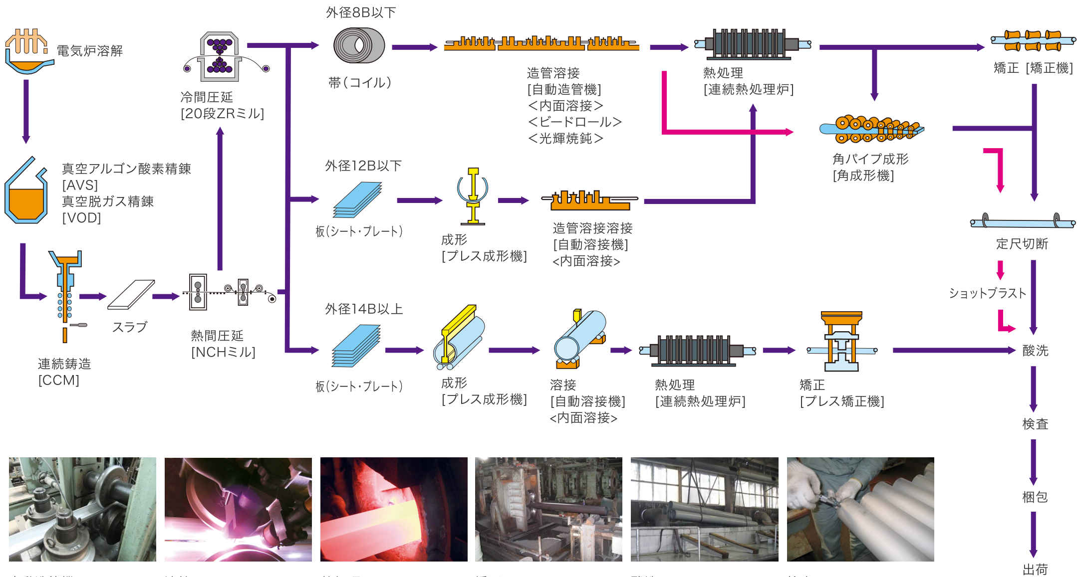
自動造管機
